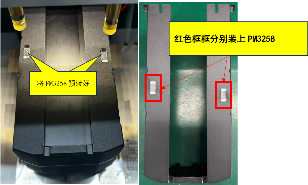
图二，将 PM3087 先放入治具，在将两个 PM3258 预装好，再进行压合，压合到位后取出检查物料无漏装或压合不到位。
