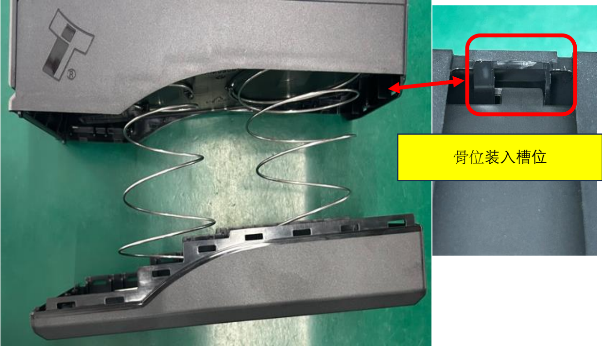
图一，将 PA3579-2 和 PA3579-5 预配在一起，注意 PM3091 的卡扣要装入上壳的槽位，上壳不能在下壳的内部。
